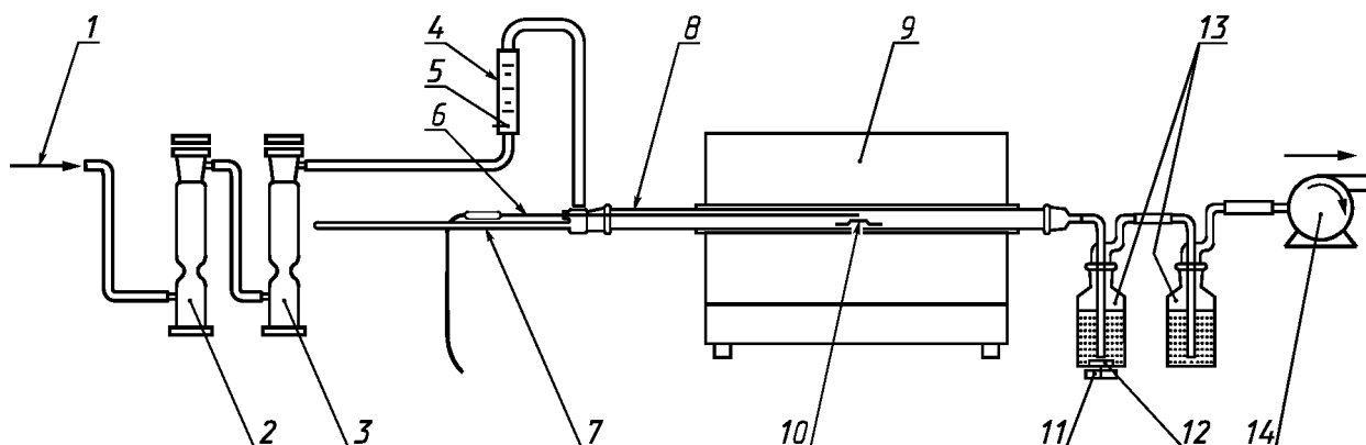
Рисунок А.4 — Оборудование для испытания по способу 2 с использованием сжатого воздуха
